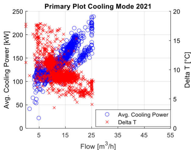
Figur 14. Flödet begränsas till det flöde som kan ge max kyleffekt. Mättnadszonen elimineras.
