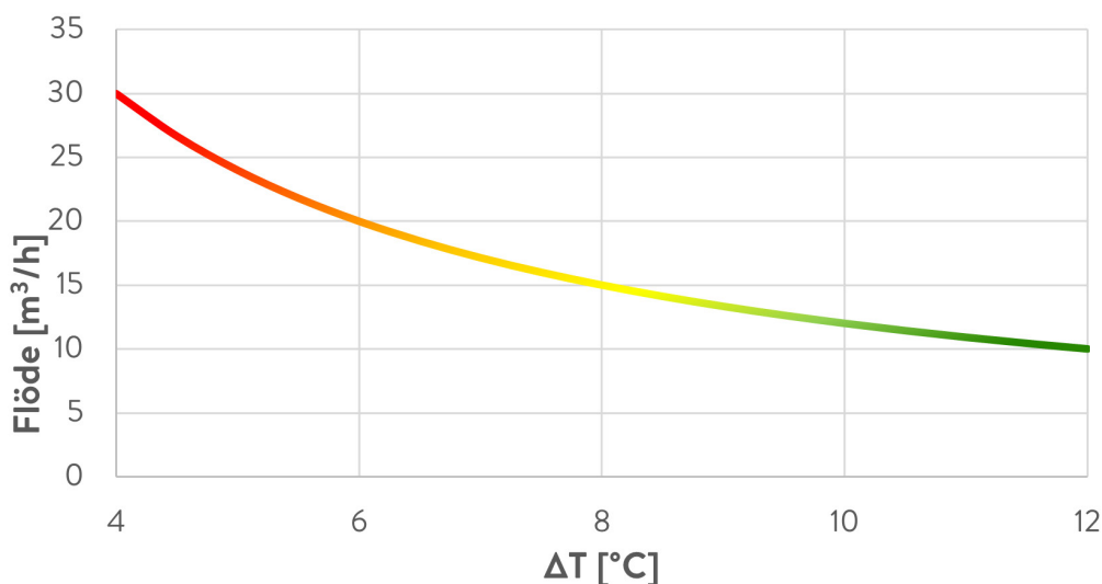
Figur 1. Potentialen för att öka \Delta T och sänka flöden är inte linjär med returtemperaturen.
