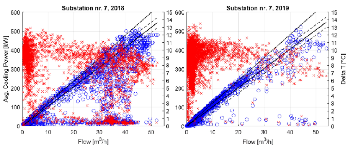
Figur 12. Exempel på fjärrkylcentral där upp till 22% besparing av max-flödet kan göras. Blå ringar motsvaras av effekt [kW] och röda kryss av \Delta T [°C] med flöde på X-axeln. Källa: Jangsten m.fl. 2022, sida 10. 1
