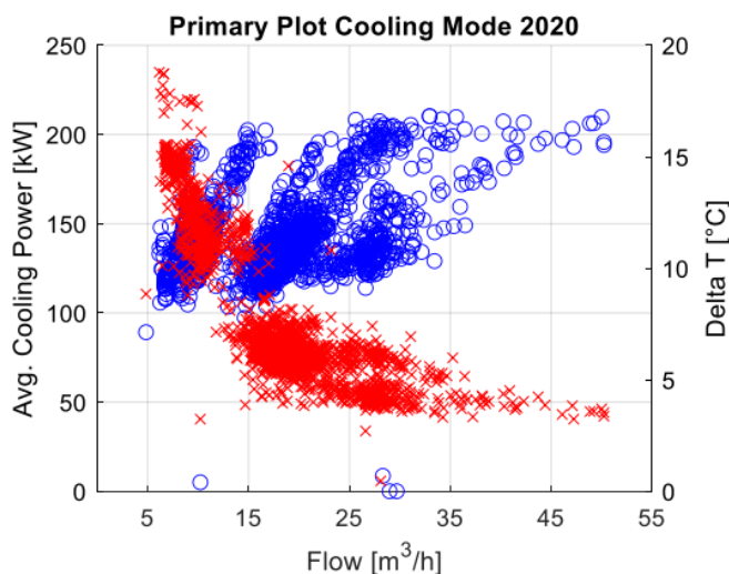
Figur 13. Maximala kyleffekt uppnås vid ca 25 m³/h. Källa: Jangsten 2022, sida 46. 2
