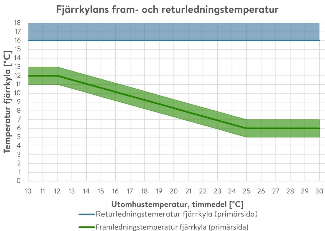
Figur 2. Framledningstemperaturen kan fluktuera och är ej konstant, men varierar också med utomhustemperaturen.
