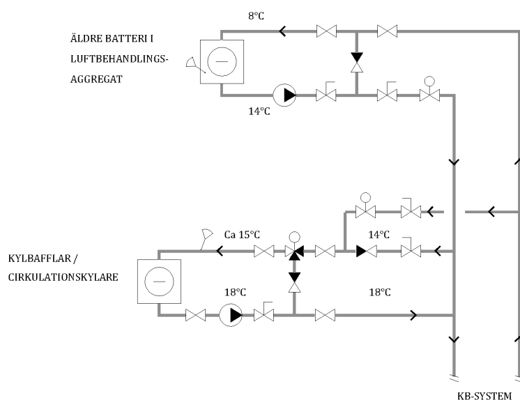
Figur 19. Kylobjekt där returledningen kopplas i serie.
