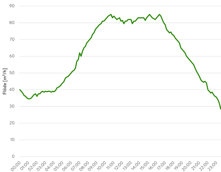
Figur 10. Exempel primärt flödesuttag vid anläggning med för stora styrventiler men som ändå fungerar tillfredställande vid större effektuttag.
