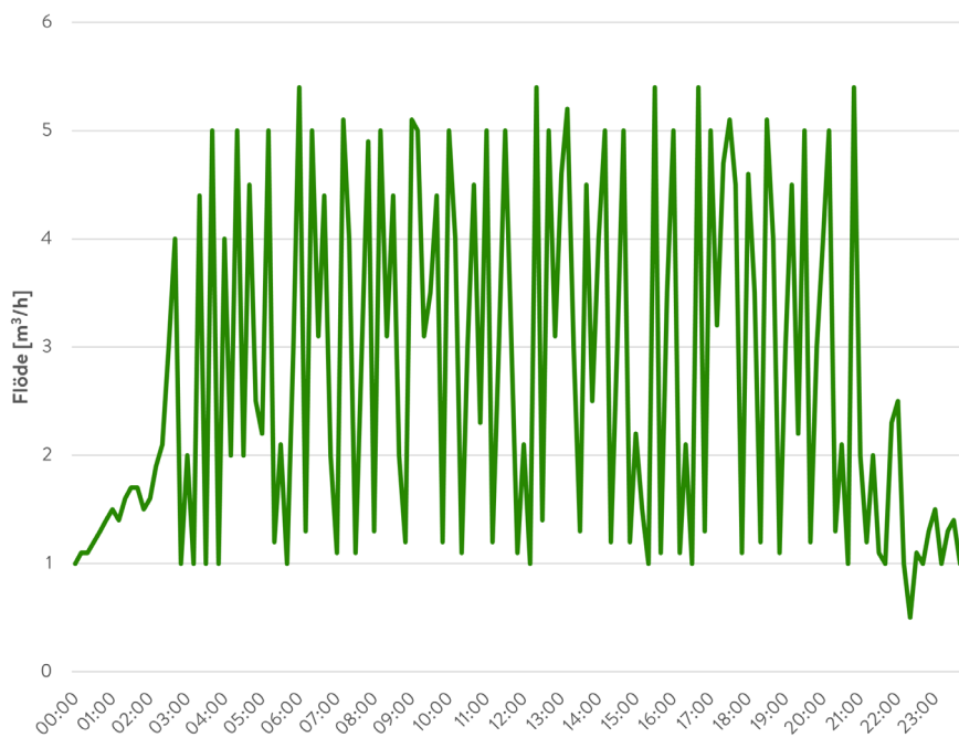
Figur 9. Exempel där primära flödet fluktuerar vid små effektuttag, med (för) stora ventiler.
