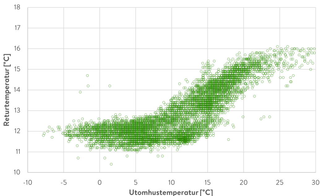
Figur 6. Exempel där returtemperaturen blir högre desto mer effektuttag som tas ut (desto högre utetemperaturen blir). Vid lägre utetemperatur shuntas mer köldbärare tillbaka via trevägsfunktionen.
