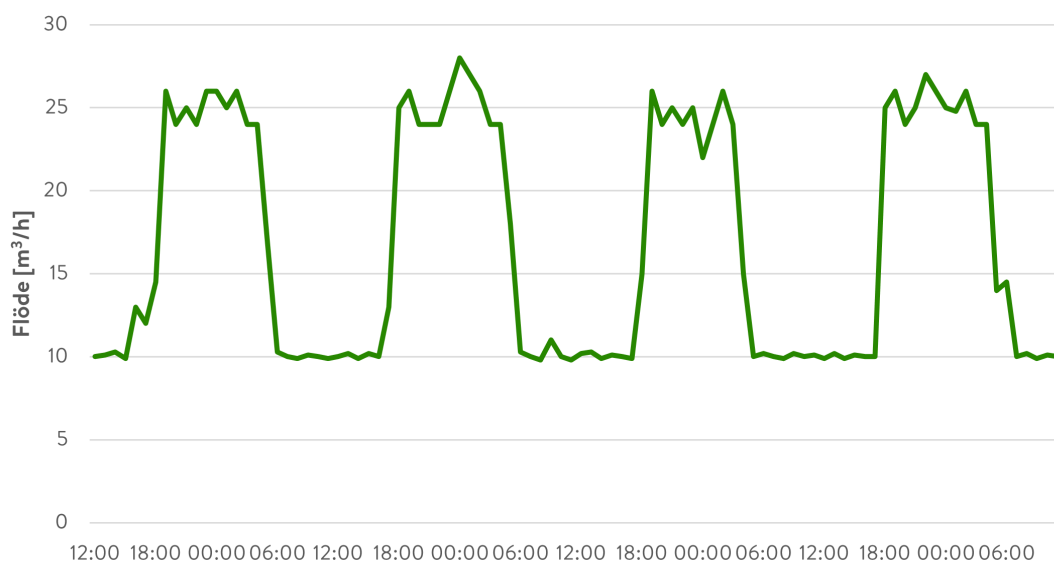
Figur 11. Exempel på ventilationsaggregatet som slås på sjunker flödet kraftigt för att sedan rätta till sig till normalt uttag.
