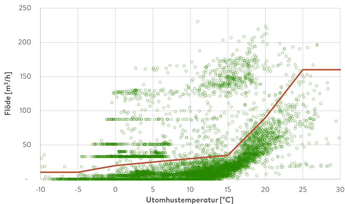
Figur 16. Flödesprofil, som fås genom att plotta flöde [ \text{m}^3/\text{h} ] och utetemperatur [ ^{\circ}\text{C} ] under ett år.
