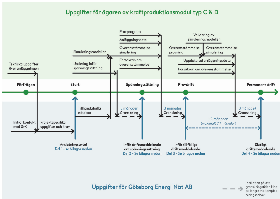
Figur 2: Process för anslutningsförfarandet av synkrona kraftproduktionsmoduler av typ C och D.
