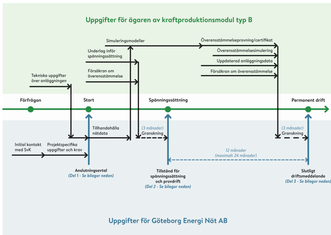
Figur 2: Process för anslutningsförfarandet av synkrona kraftproduktionsmoduler av typ B
